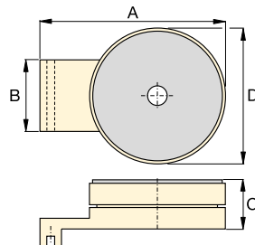
Placa giratoria ES-60, ES-80
