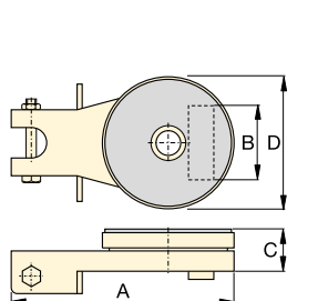
Placa giratoria ES-1, ES-10, ES-15, ES-30
