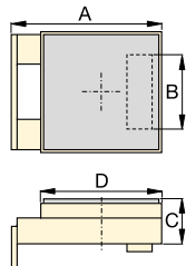
Placa fija ELP-10, ELP-15, ELP-30
